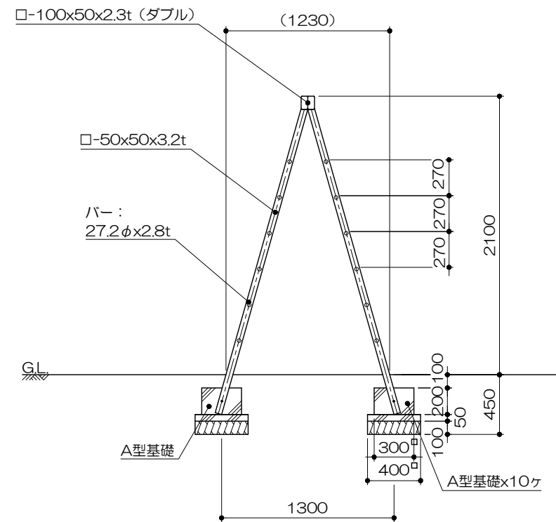
側面図 S= 1 : 40
