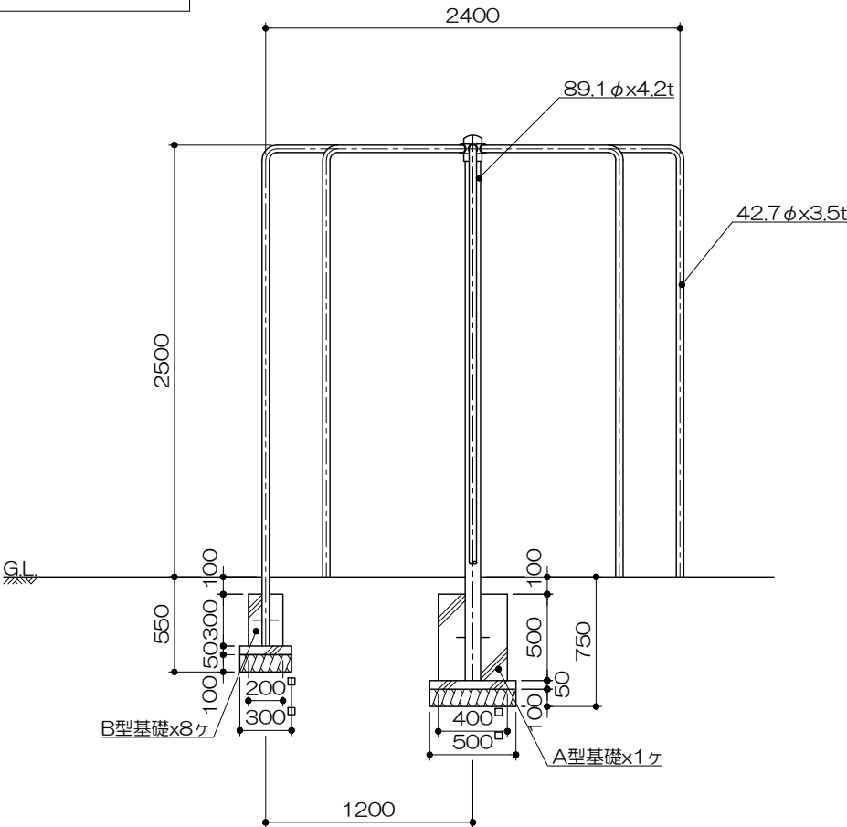
立面図 S= 1 : 40
