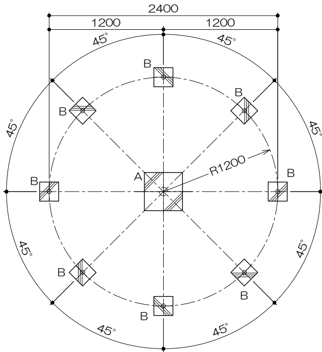
基礎平面図 S= 1 : 40
