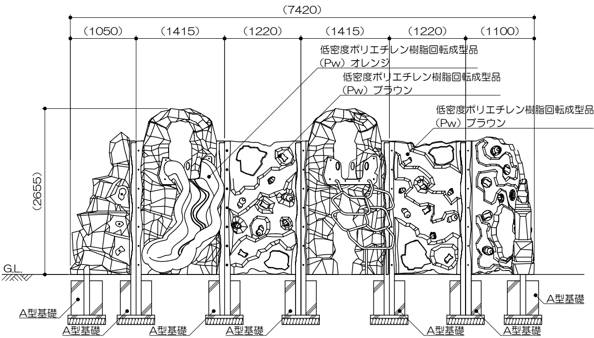
立面図 S= 1 : 60
