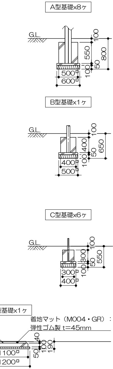
基礎リスト S= 1 : 60
