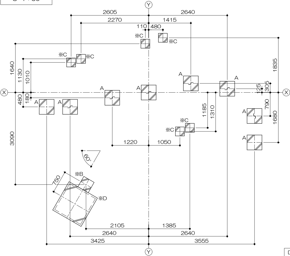
PG31-CL008+マット付 ロックブロック (5) S=図示 (D)
