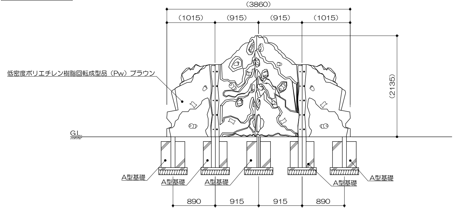
立面図 S= 1 : 50
