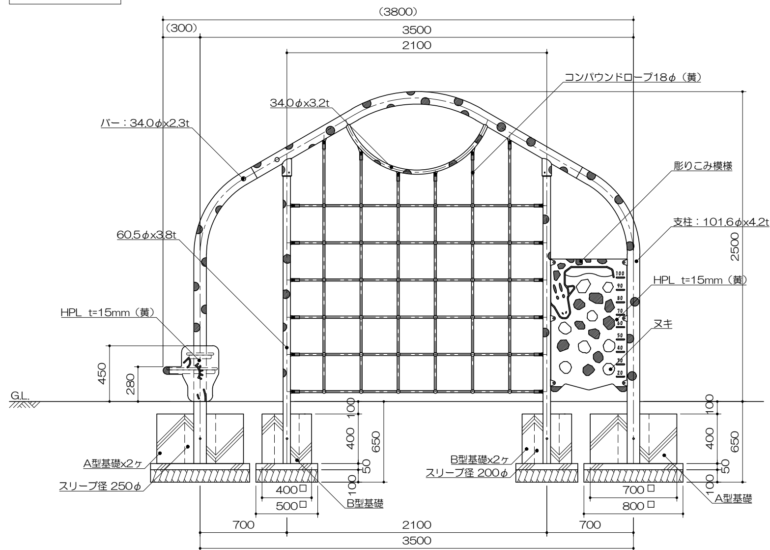
立面图
