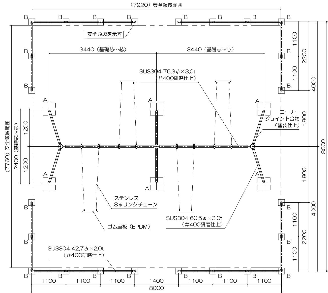
立面図 S= 1 : 60
