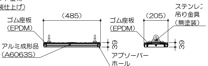
ゴム座板断面図 S= 1 : 20
