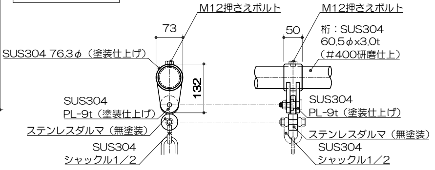
側面図 S= 1 : 60
