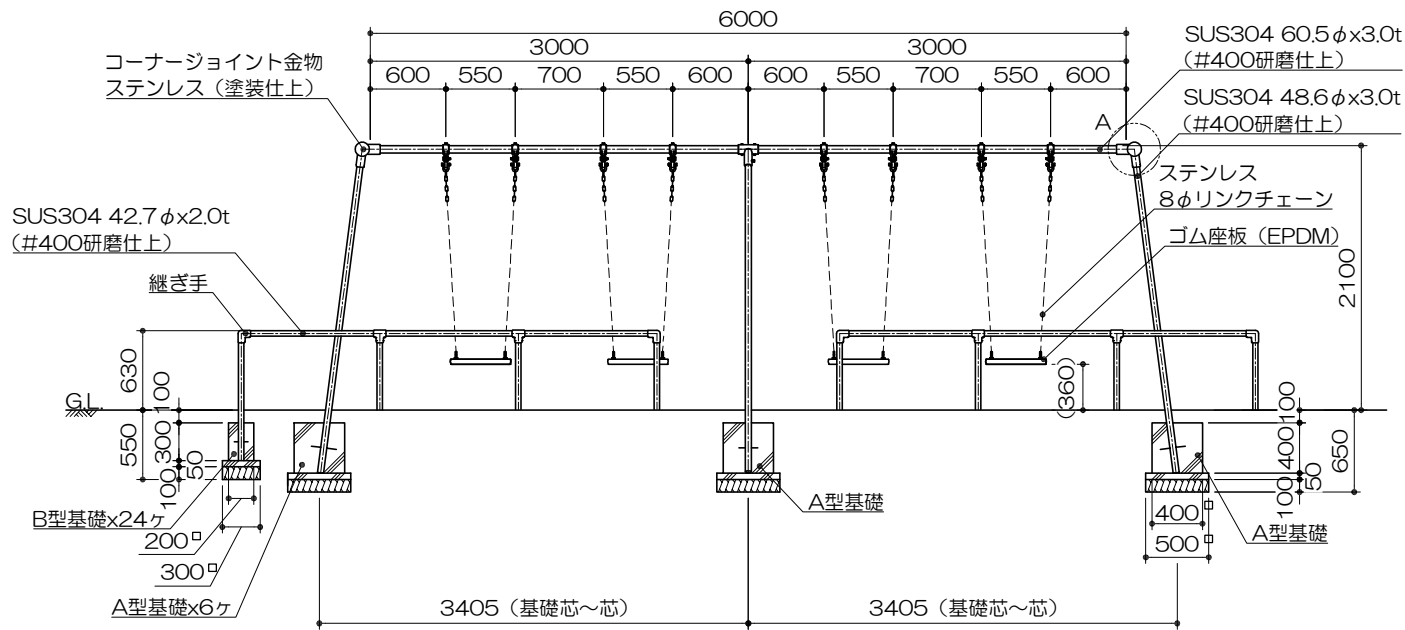
立面図 S= 1 : 60
