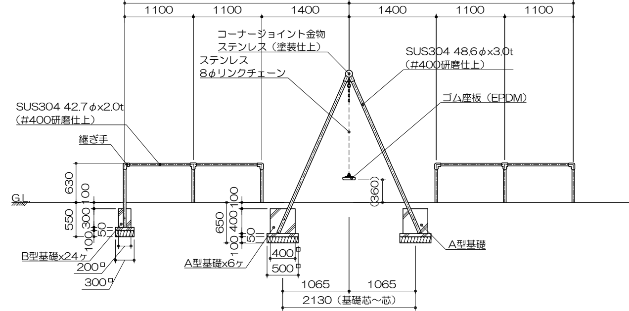
側面図 S= 1 : 60
