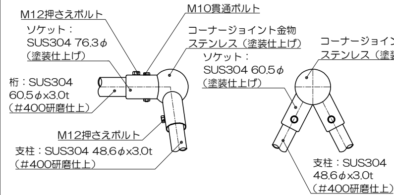
ブランコハンガー詳細図 S= 1 : 10
