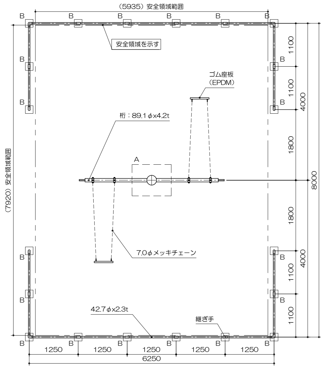
平面図 S= 1 : 60
