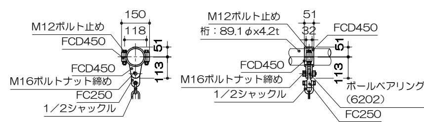
側面図 S= 1 : 60
