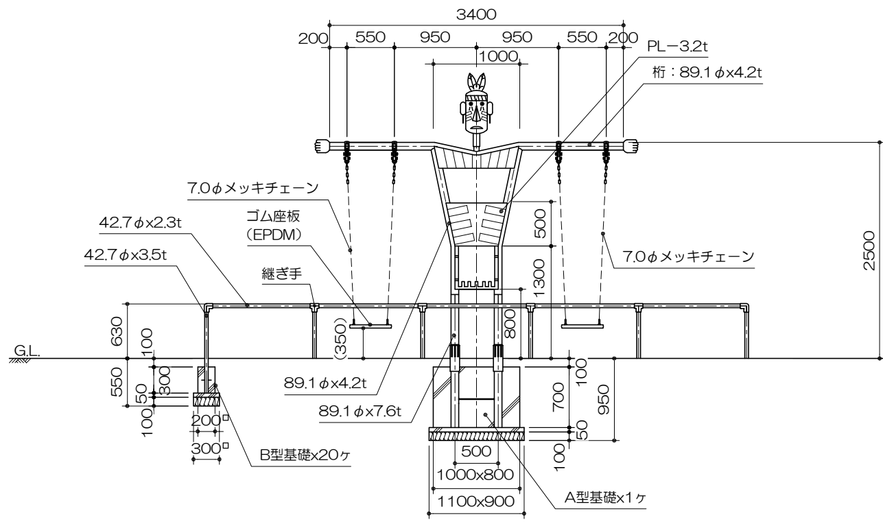
立面図 S= 1 : 60
