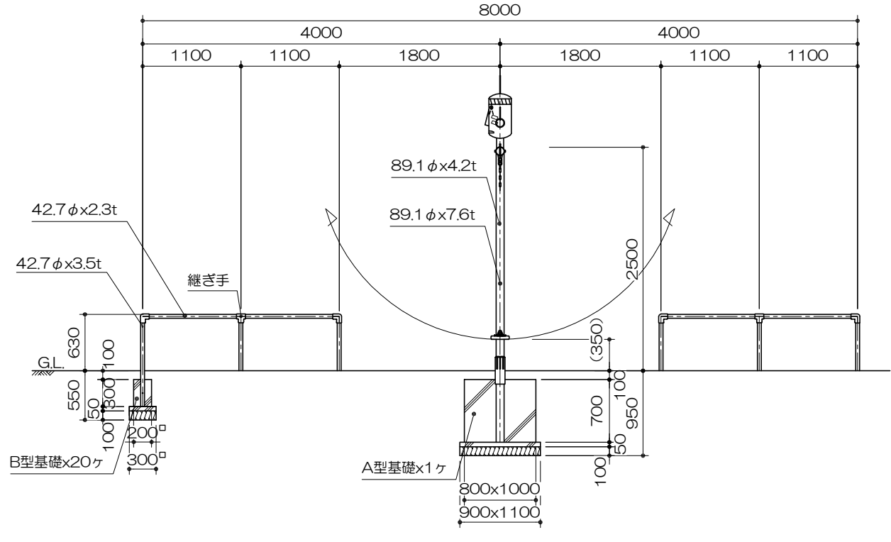
側面図 S= 1 : 60
