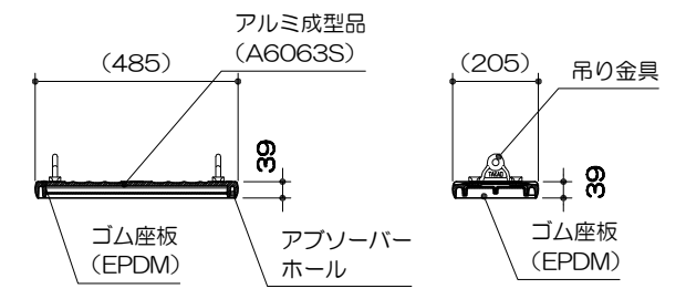
ゴム座板断面図 S= 1 : 20
