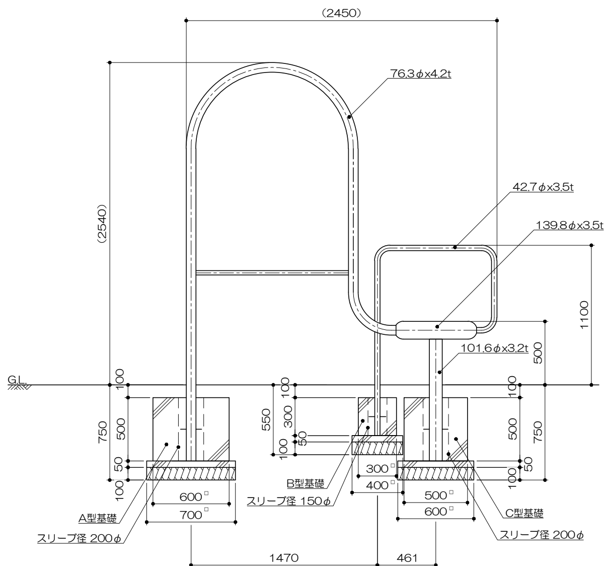
立面図 S= 1 : 30
