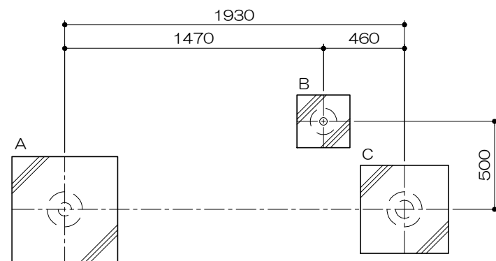
基礎平面図 S= 1 : 30
