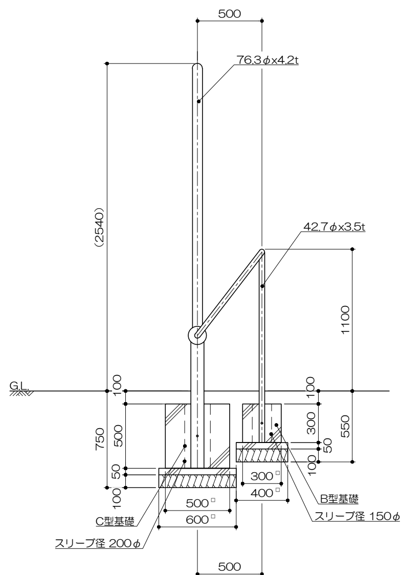
側面図 S= 1 : 30
