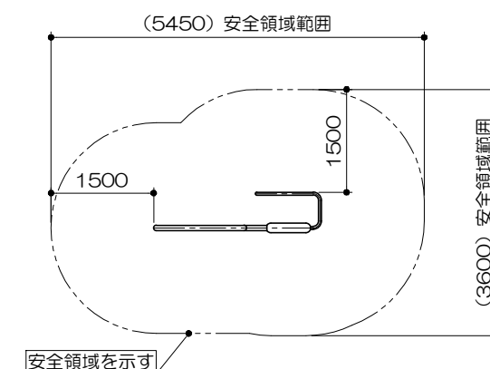
安全領域範囲 S= 1 : 100
