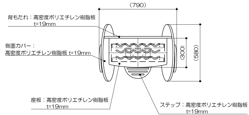
平面図 S= 1 : 20
