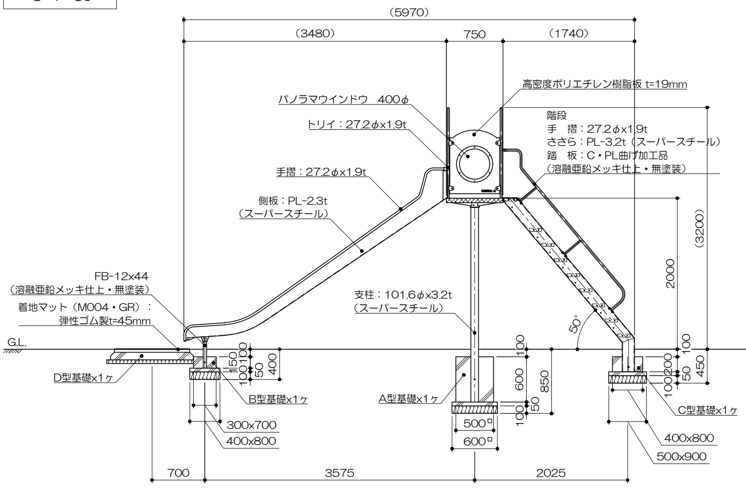
立面図 S= 1 : 50
