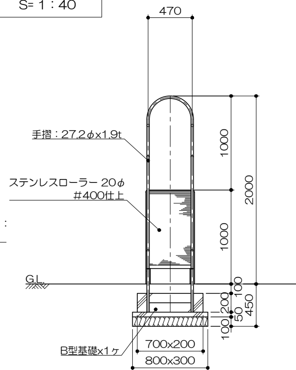
側面図 S= 1 : 40
