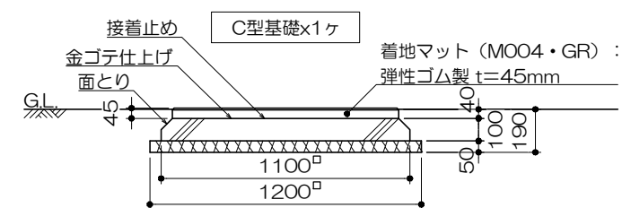
C型基礎詳細図 S= 1 : 30
