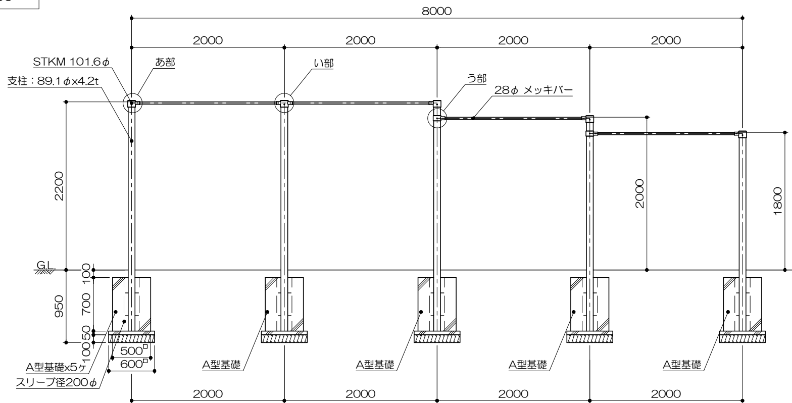
立面図 S= 1 : 50
