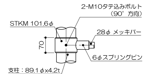
う部詳細図 S= 1 : 10
