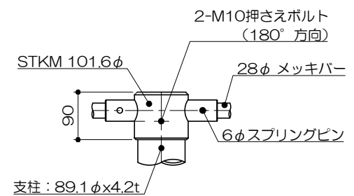
う部詳細図 S= 1 : 10
