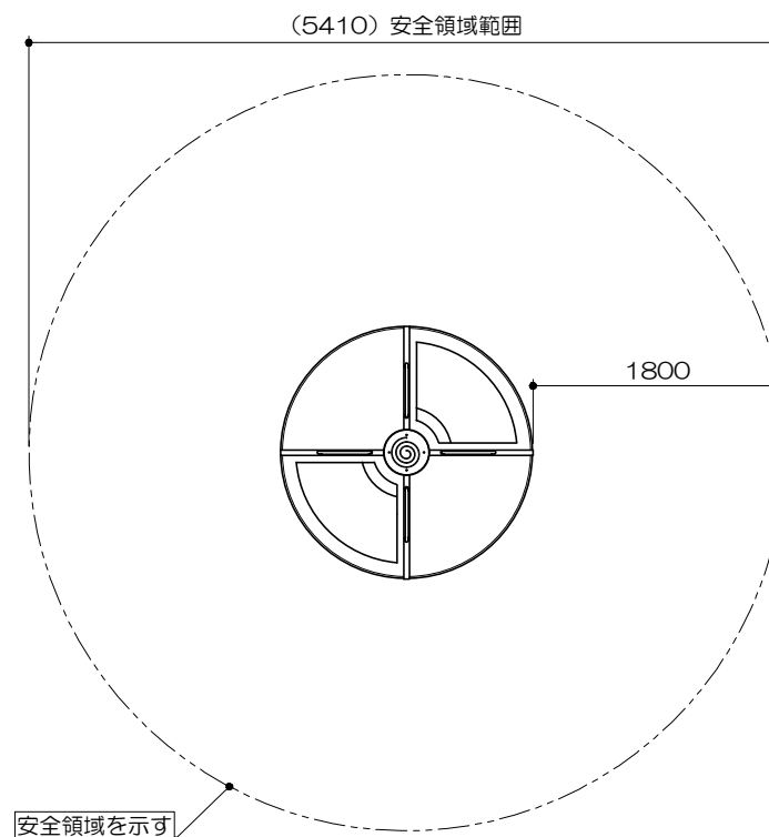
安全領域範囲 S= 1 : 60
