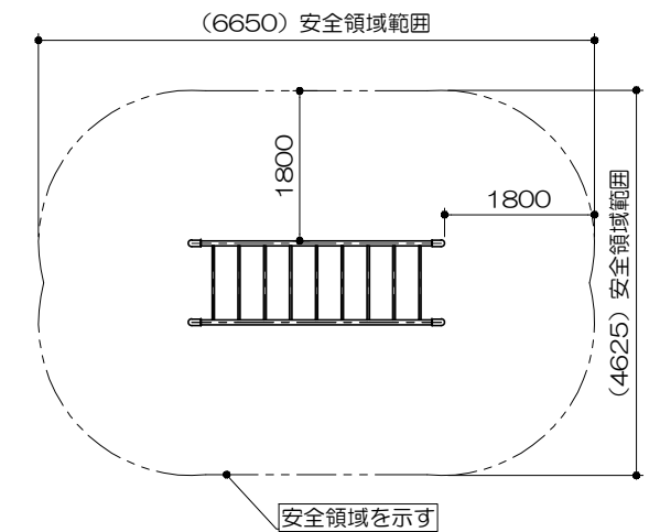
安全領域範囲 S= 1 : 100
