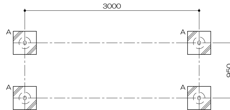
基礎平面図 S= 1 : 40
