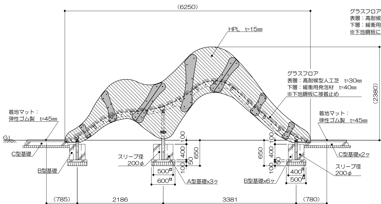
立面図 S= 1 : 50
