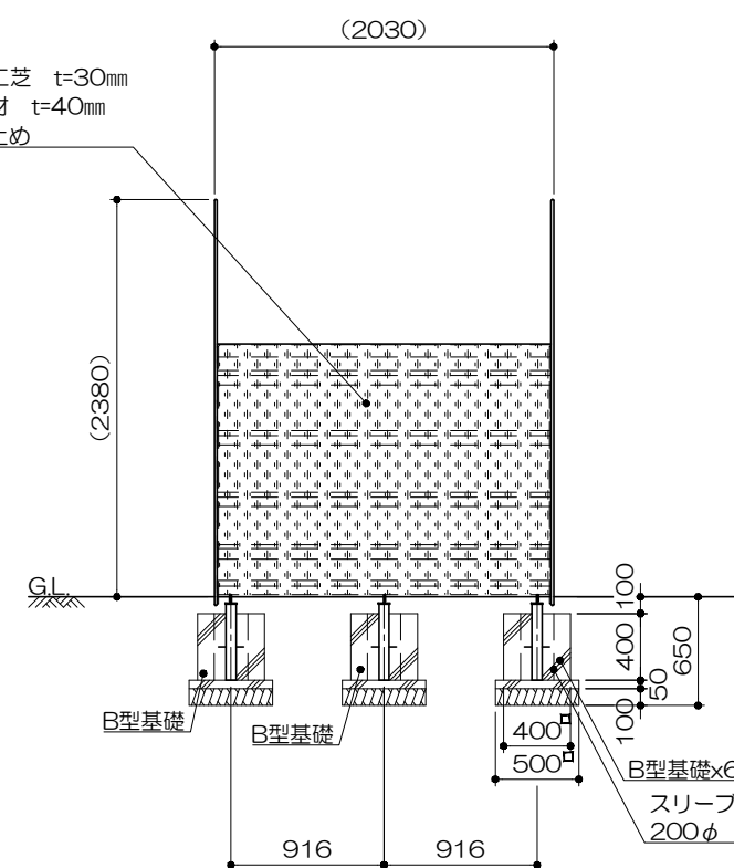
側面図 S= 1 : 50
