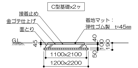
C型基礎詳細図 S= 1 : 50
