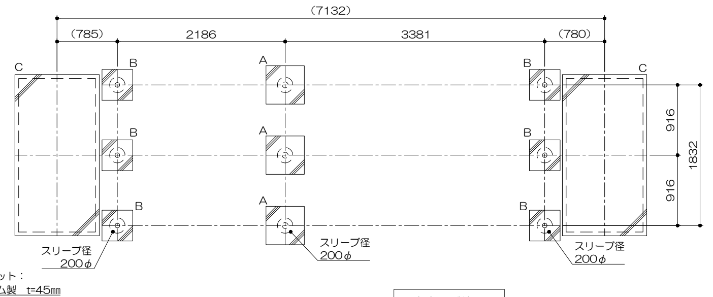
安全領域範囲 S= 1 : 200
