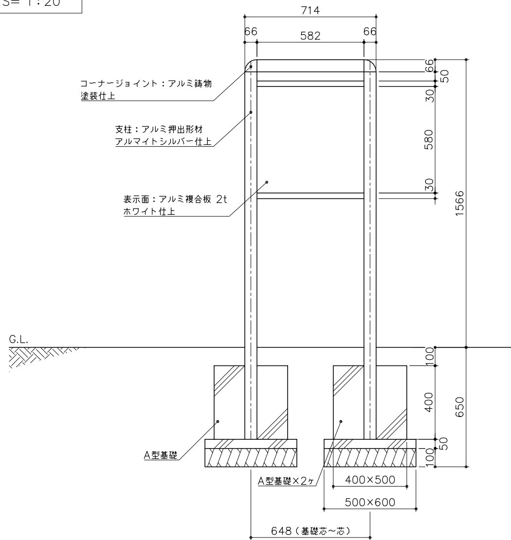
立面図 S= 1:20
