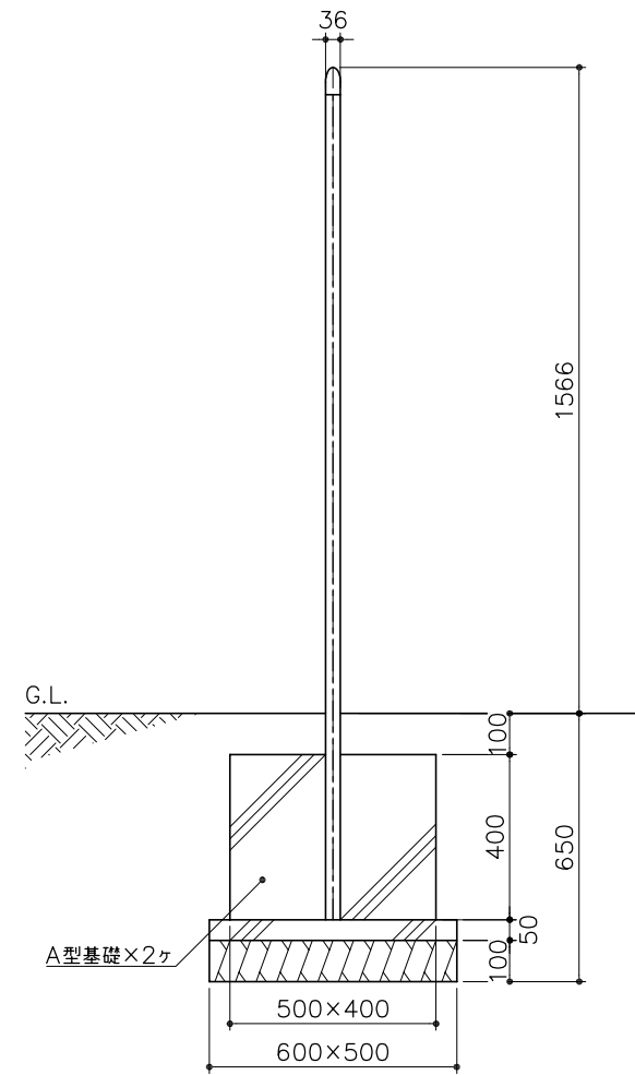
側面図 S= 1:20
