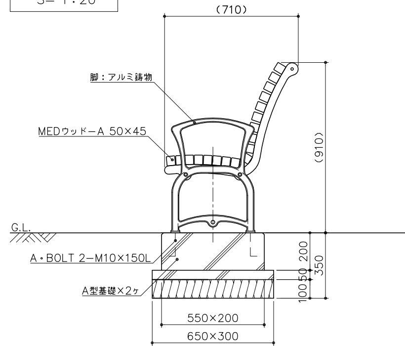
側面図 S= 1:20
