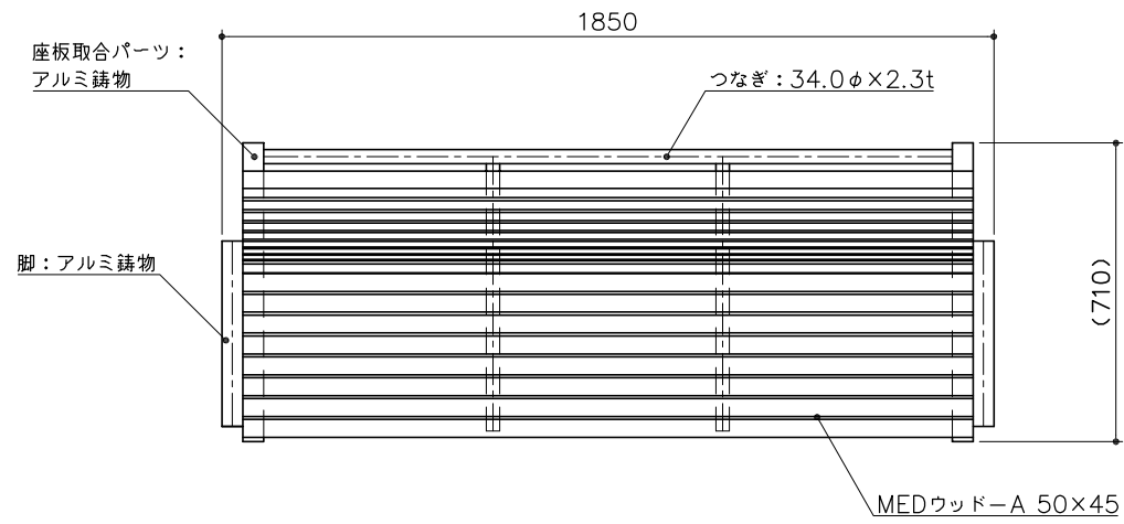
平面図 S= 1:20
