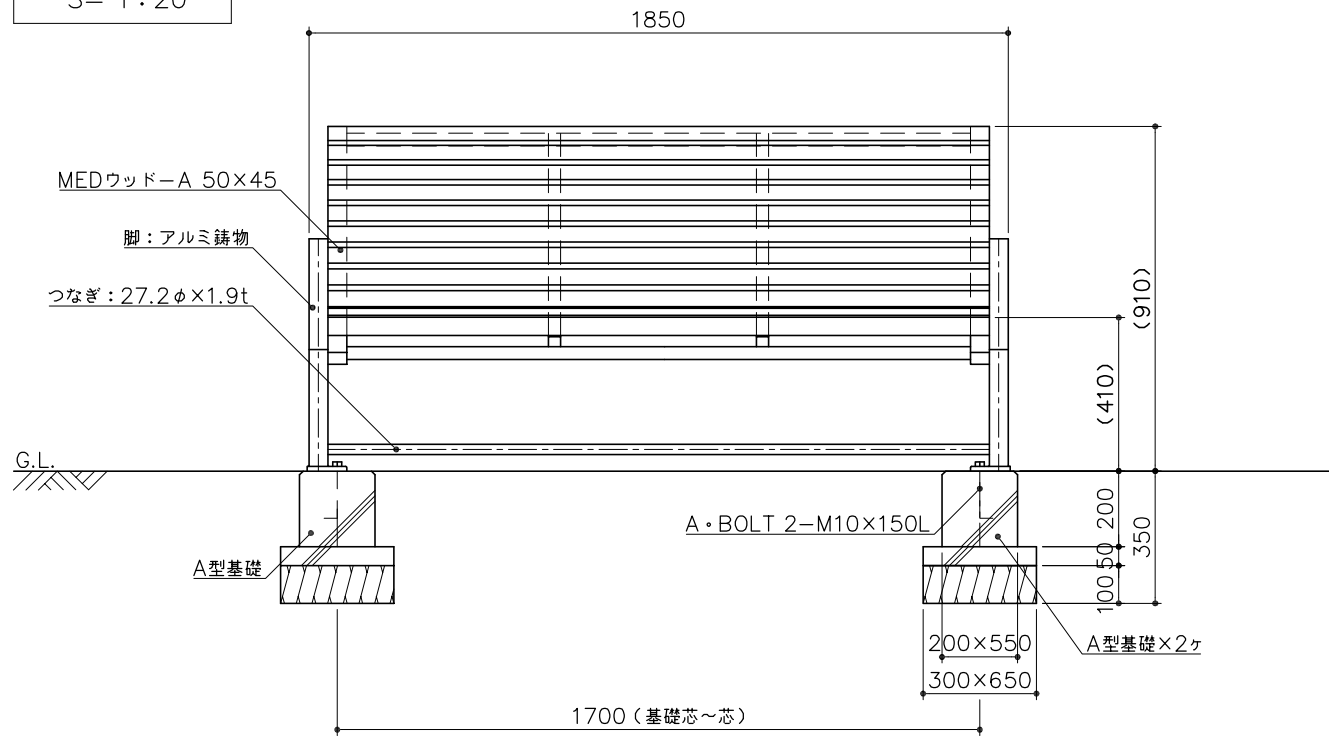
立面図 S= 1:20
