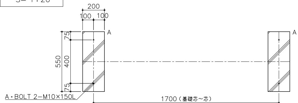
基礎平面図 S= 1:20
