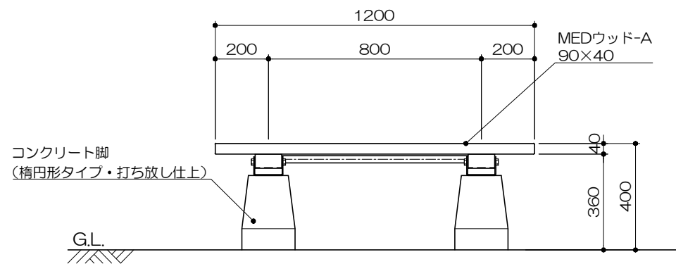
立面図 S= 1 : 20
