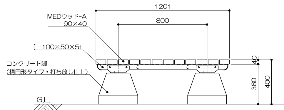
側面図 S= 1 : 20
