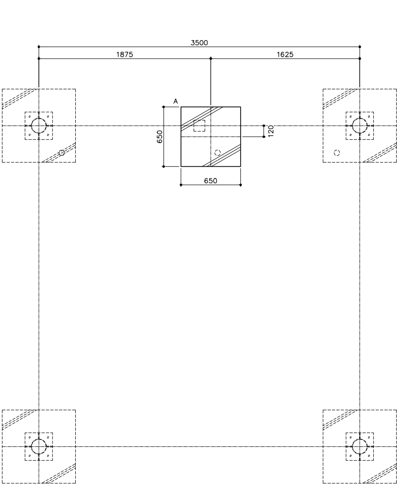
基礎平面図 S= 1:20
