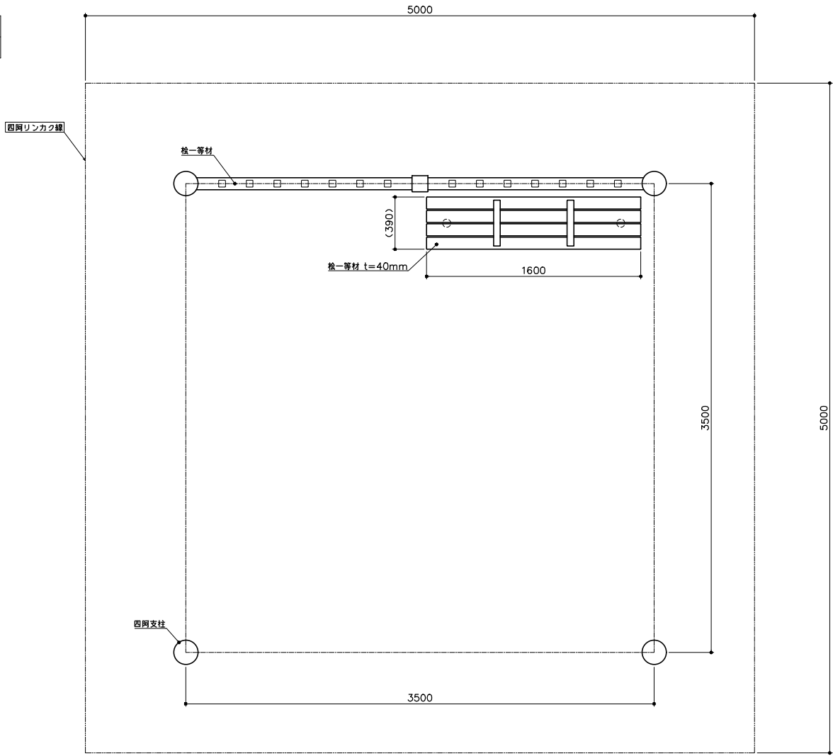
平面図 S= 1:20
