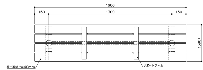
ベンチ平面図 S= 1:10
